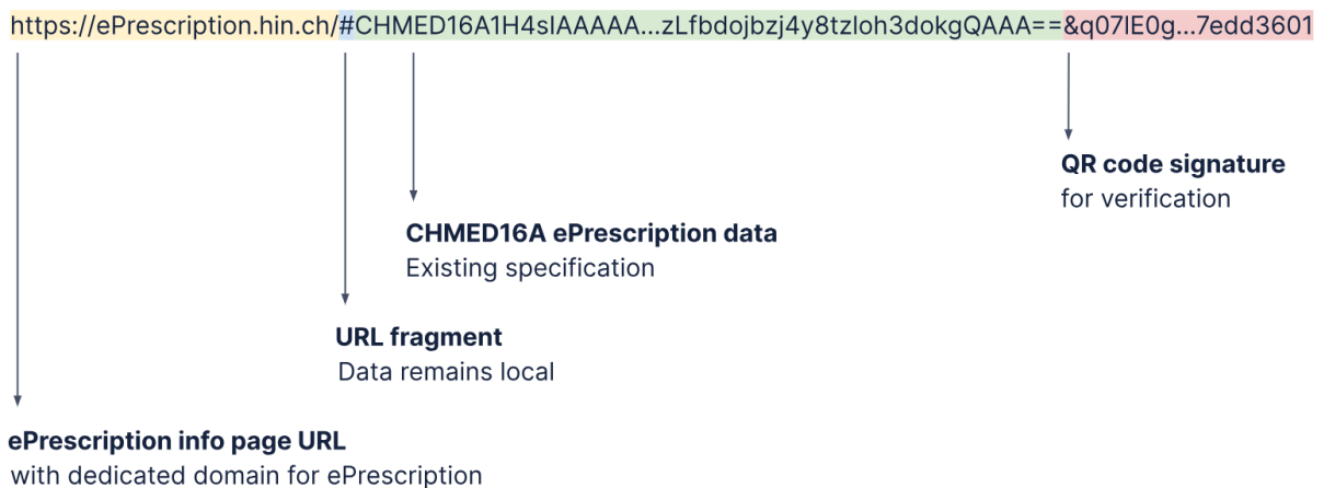
Abbildung 4: Aufbau des E-Rezepts inklusive Signatur
