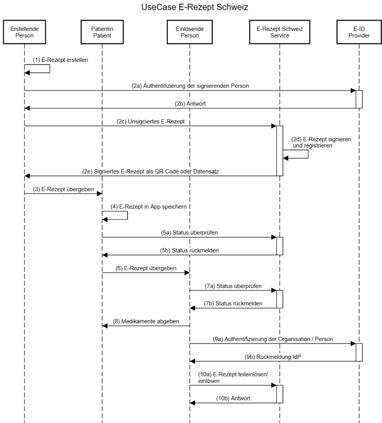
Abbildung 6: Sequenzdiagramm für den kompletten UseCase E-Rezept
